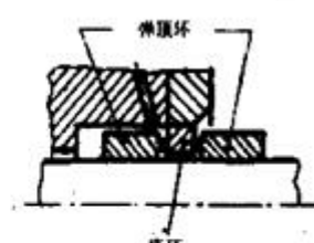
D3 面对面配置 (有旋转密封环 (配合环)也可同样配置)
