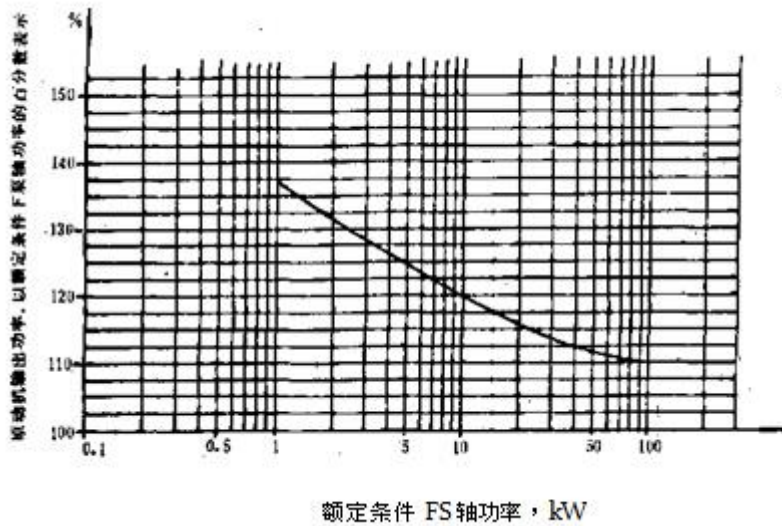
图 2 以额定条件下的泵轴功率的百分数表示的原动机输出功率 对于不确定的工作条件：作为共轴式泵的驱动机的原动机，其额定输出功率必须满足安装的给定直径叶轮在任何工作条件下功率需求。这些情况下不再需要额外余量。
