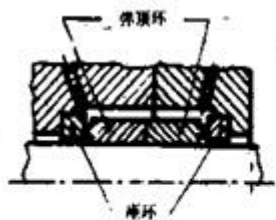
D1 背靠背配置，
